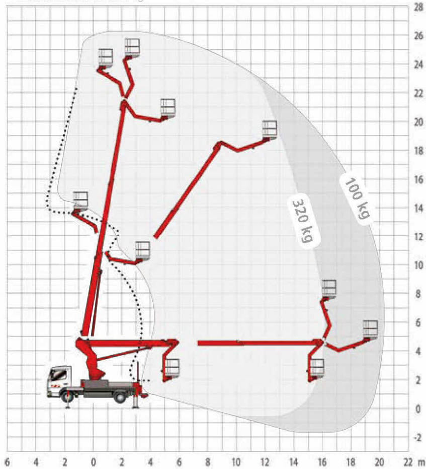
Arbeitskorblast bis 320 kg
